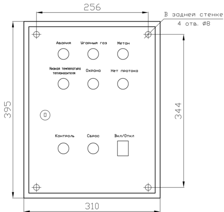
Габаритные и установочные размеры блока АО-20.05Рд
