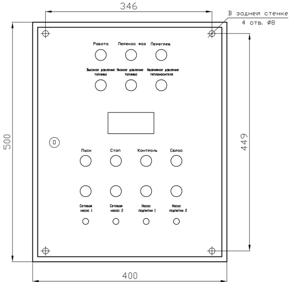
Габаритные и установочные размеры блока АО-20.05Р
