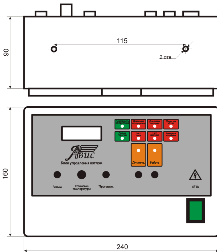
Габаритные и установочные размеры блока АК-00(04).10
